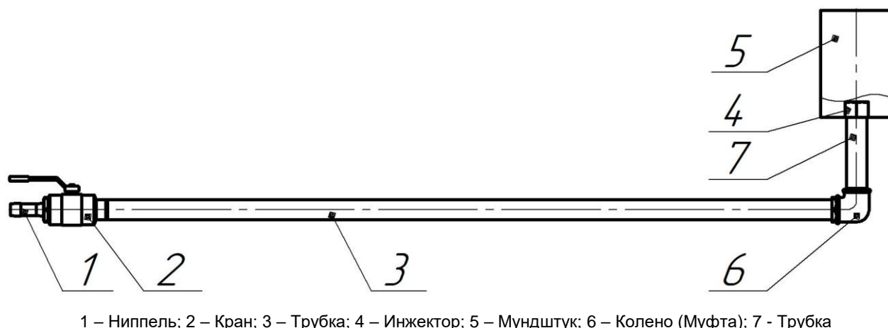
Рисунок 1 – Горелка МП-ГПМИ
