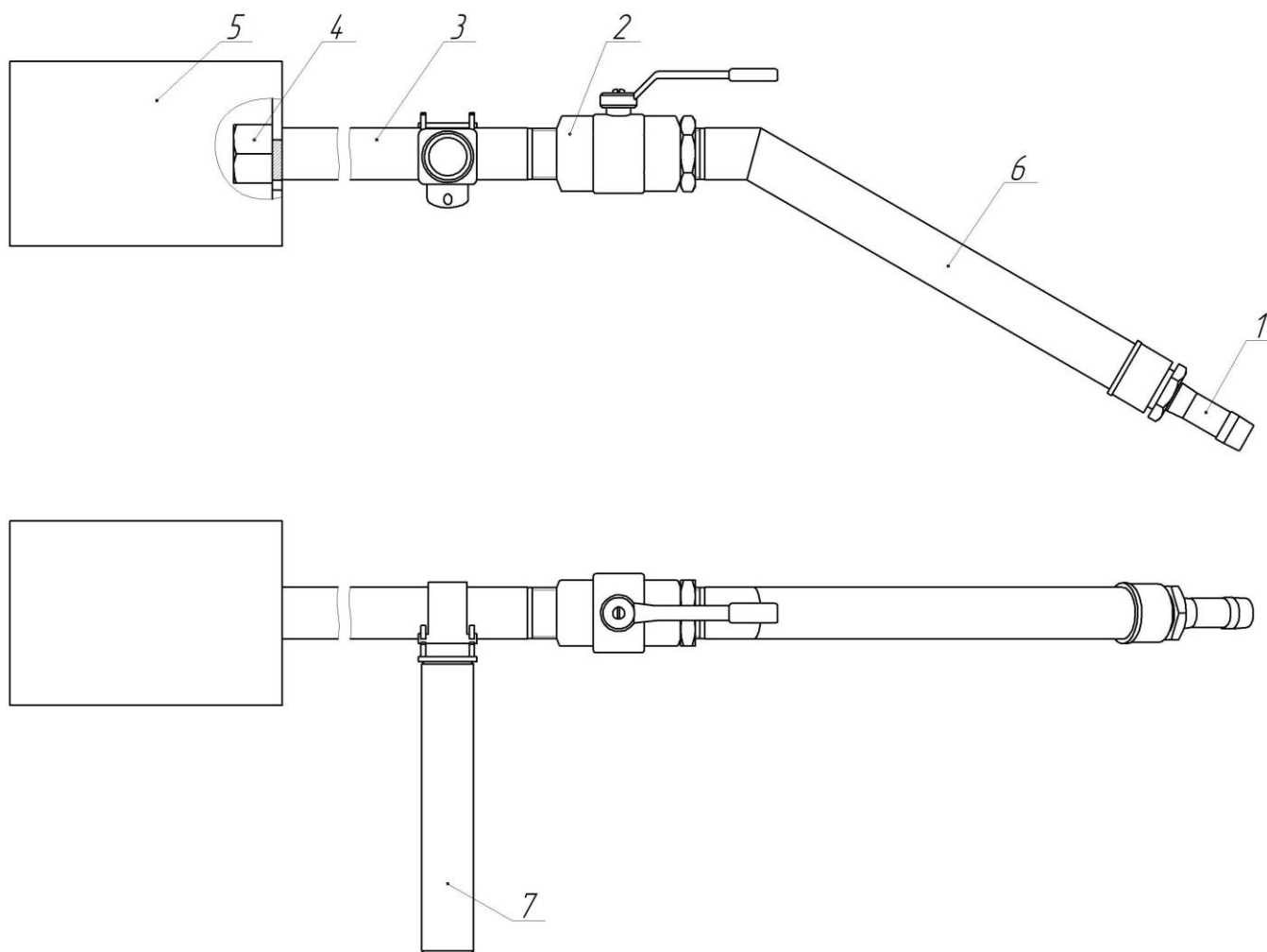
Рисунок 1 – Горелка МП-ГПМИ-2
